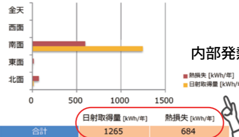
暖房期の窓からの日射取得量と熱損失 内訳
